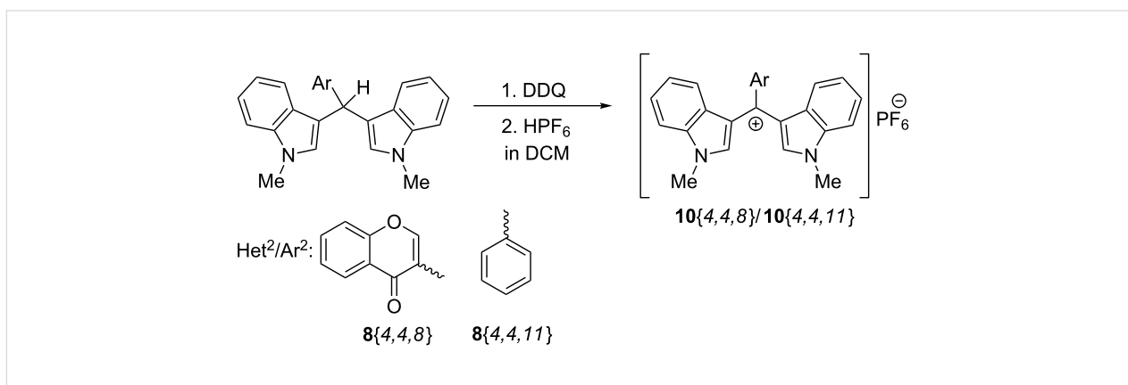
Scheme 8: Synthesis of crowded (Het 1 2 Het 2 /Ar 2 )C + PF 6 − salts 10 .
